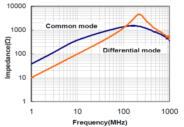
CM7060FBQ1 -132
