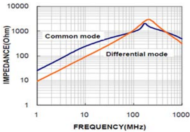
CM7060FBQ1 -102
