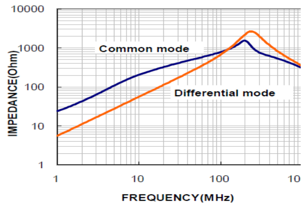
CM7060FBQ1-701
