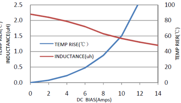
PIC05030-2R2M
