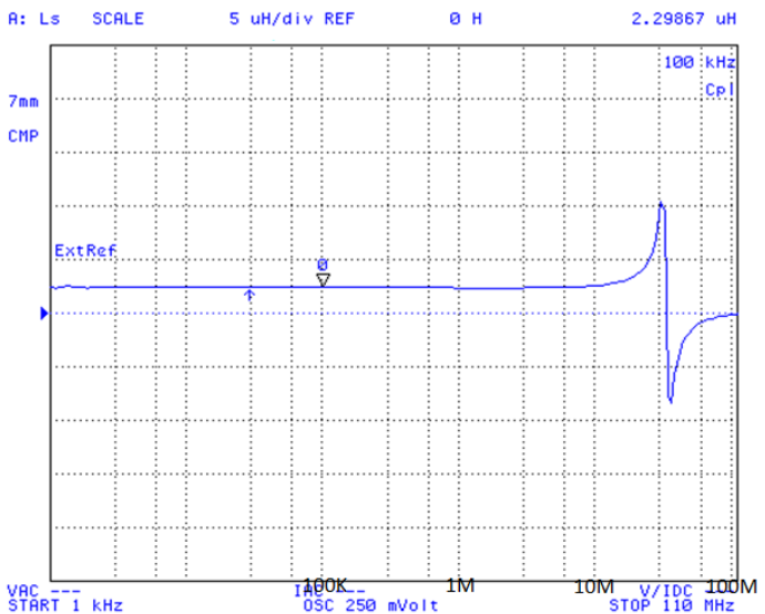
PI07018-2R2M
