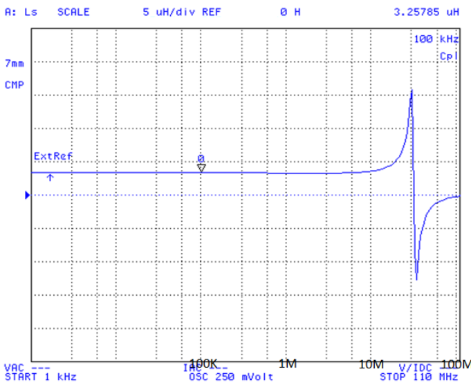
PI07018-3R3M
