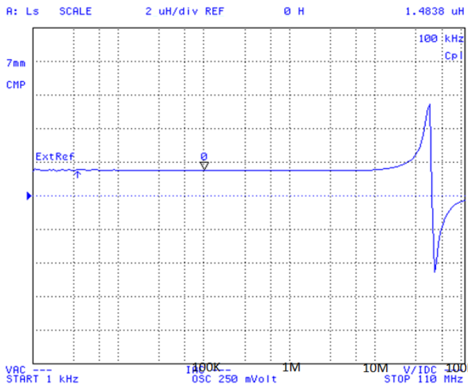
PI07018-1R5M
