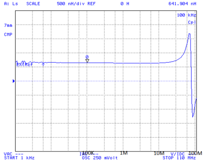
PI07018-1R0M
