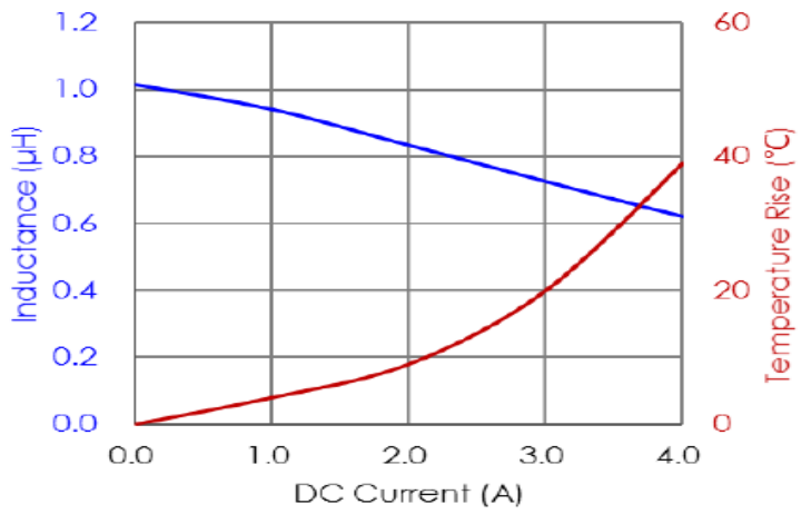
PIC252012-1R0
